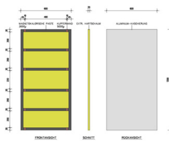
INFRAROT-DECKENPLATTE TYP. 1, M. 1:10 ALLE MAßE IN MM
